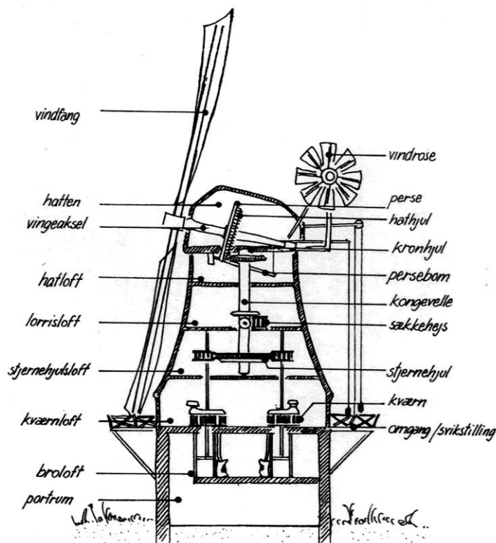
Skematisk tegning af en gallerihollænder med lofter og vingefang. Jens Kortermann Larsen.
